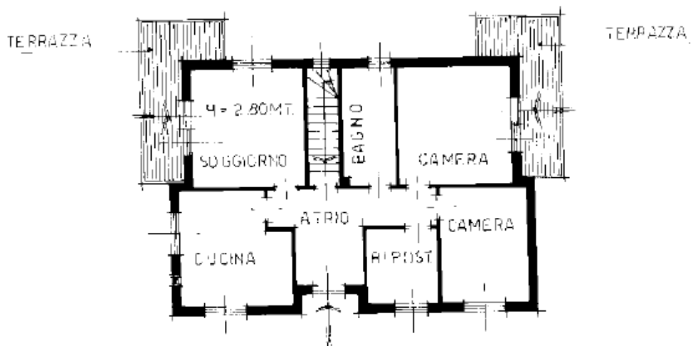
PIANTA PIANO TERRA RIALZATO
